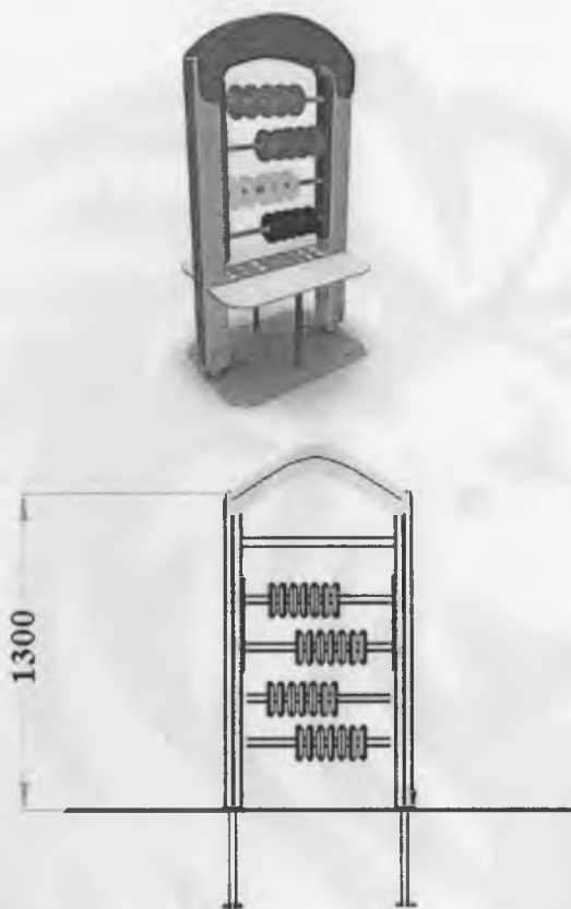
Рисунок 1 - Схема сборки (Изделие поставляется в собранном виде)
